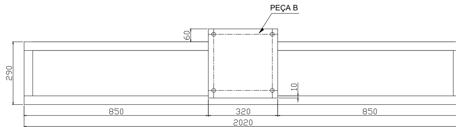
SEÇÃO CC DETALHE DA MONTAGEM DA PEÇA B NA ESTRUTURA
