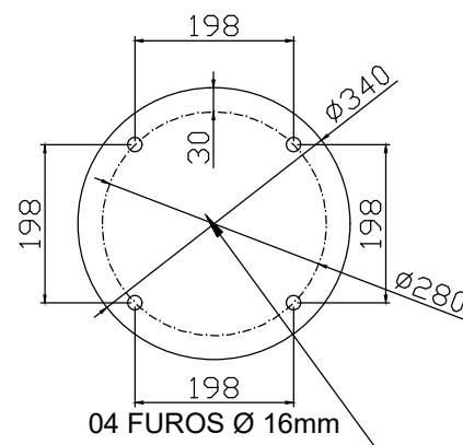
CHAPA GABARITO
