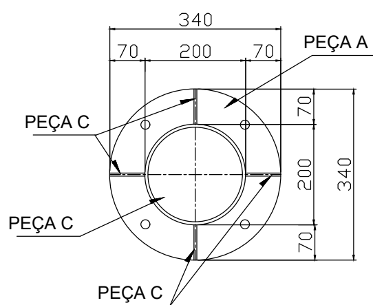
SEÇÃO AA
