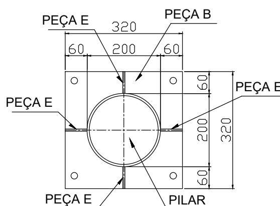
SEÇÃO BB
